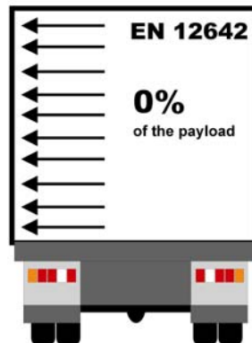
Joonis 12: Tentautode külgsentele esitatavad tugevusnõuded
