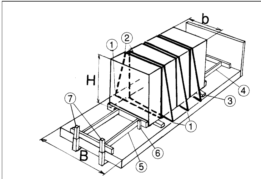
Joonis 72: Silmussidemete ja tõkistega kinnitatud suur üksus külgluukideta platvormil
