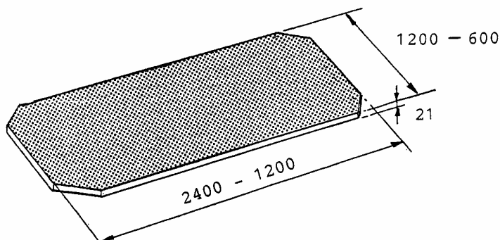
Joonis 48 Vahelaud:
