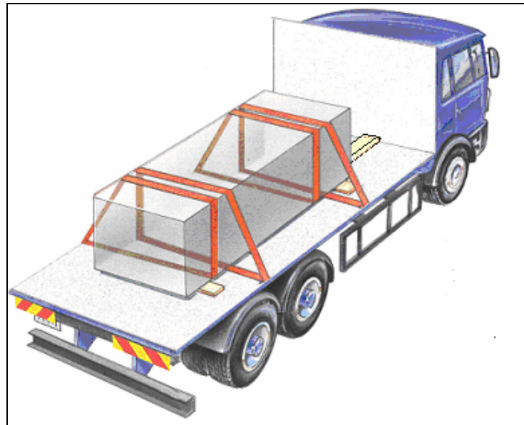
Joonis 29: Silmusside
