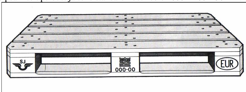
Joonis 62: Euroalus
