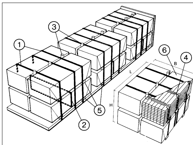
Joonis 77: Kokkupakitud saematerjal tasapinnalisel keskmiste vertikaaltugedega veoplatvormil
